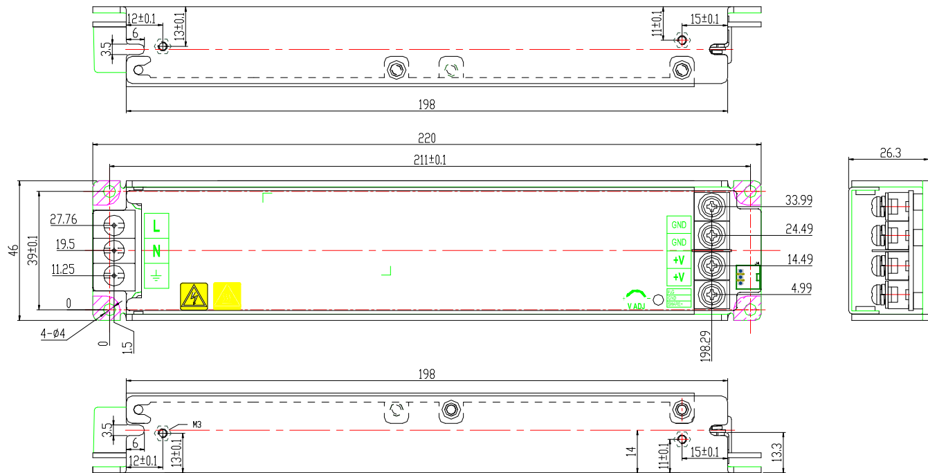
外形尺寸及安装孔——端子坐标图
